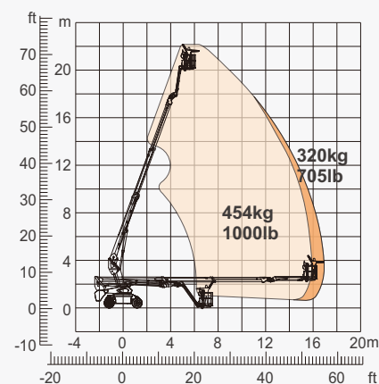
Bewegungsbereich
