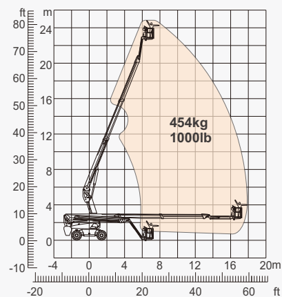
Bewegungsbereich
