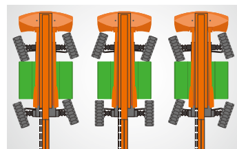
Mehrere Lenkungsmodi
